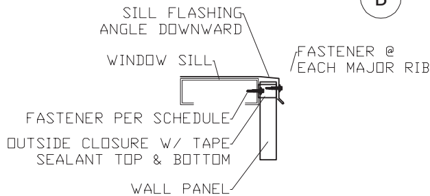
C DOOR / WINDOW SILL
