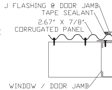
B DOOR / WINDOW JAMB
