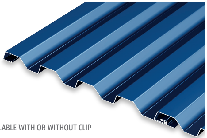
FASTENER FLANGE
