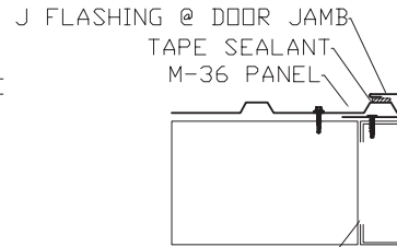
B DOOR / WINDOW JAMB
