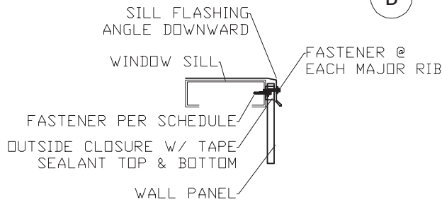
C DOOR / WINDOW SILL
