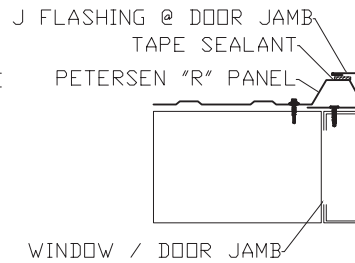
B DOOR / WINDOW JAMB
