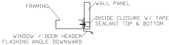
A DOOR / WINDOW HEADER
