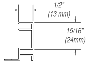
CRAX-10 EXTRUSION
