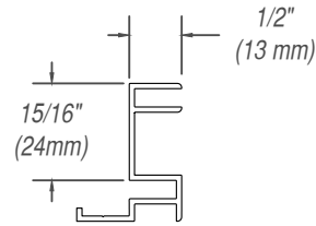
CRAX-11 EXTRUSION
