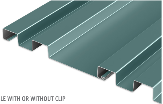
FASTENER FLANGE
