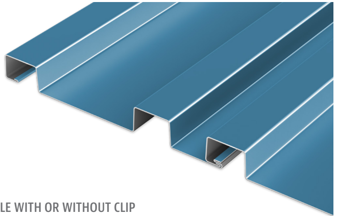
FASTENER FLANGE
